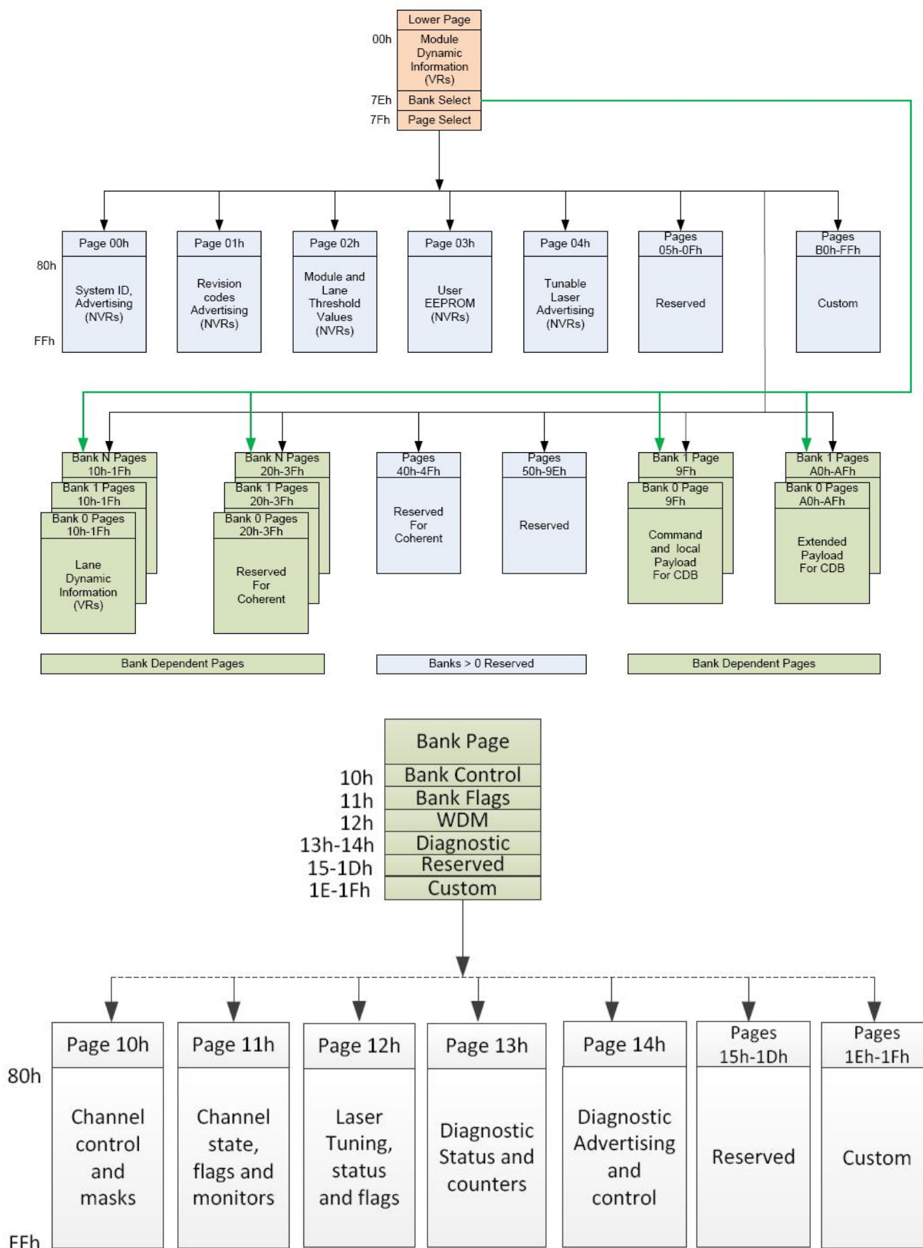
Figure4. QSFP DD Memory Map
